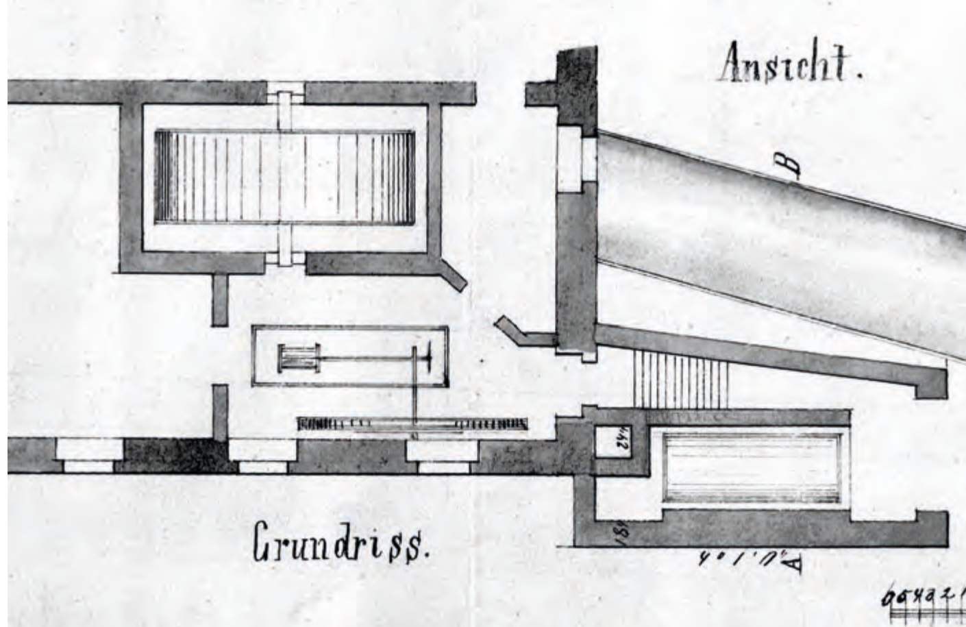
Nahoře: Kotle pro parní stroje v Preibischově továrně v Dětrichově Dole: Valcha u Věže v Liberci; parní stroje se často kvůli transmisním rozvodům instalovaly v blízkosti starších vodních kol
