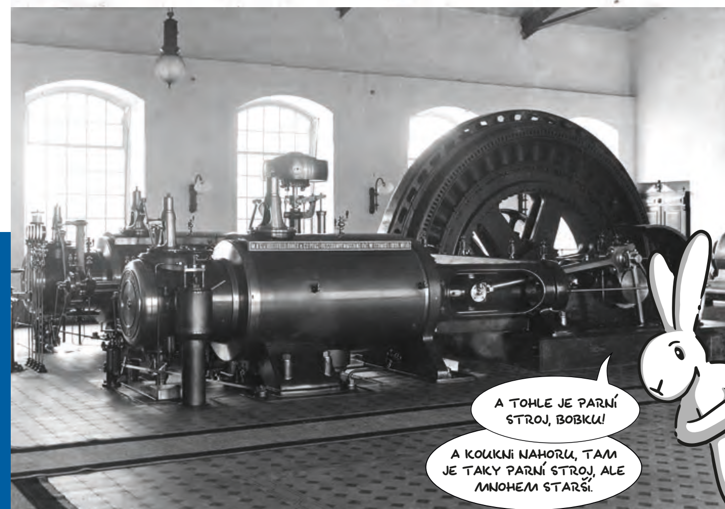
Nahoře: Jeden z nejstarších náčrtů parního stroje v Liberci; pochází asi z 60. let 19. století, měl výkon několika koní a sloužil v železničních opravnách Dole: Parní stroj spřažený s velkým dynamem v Liberci na počátku 20. století
