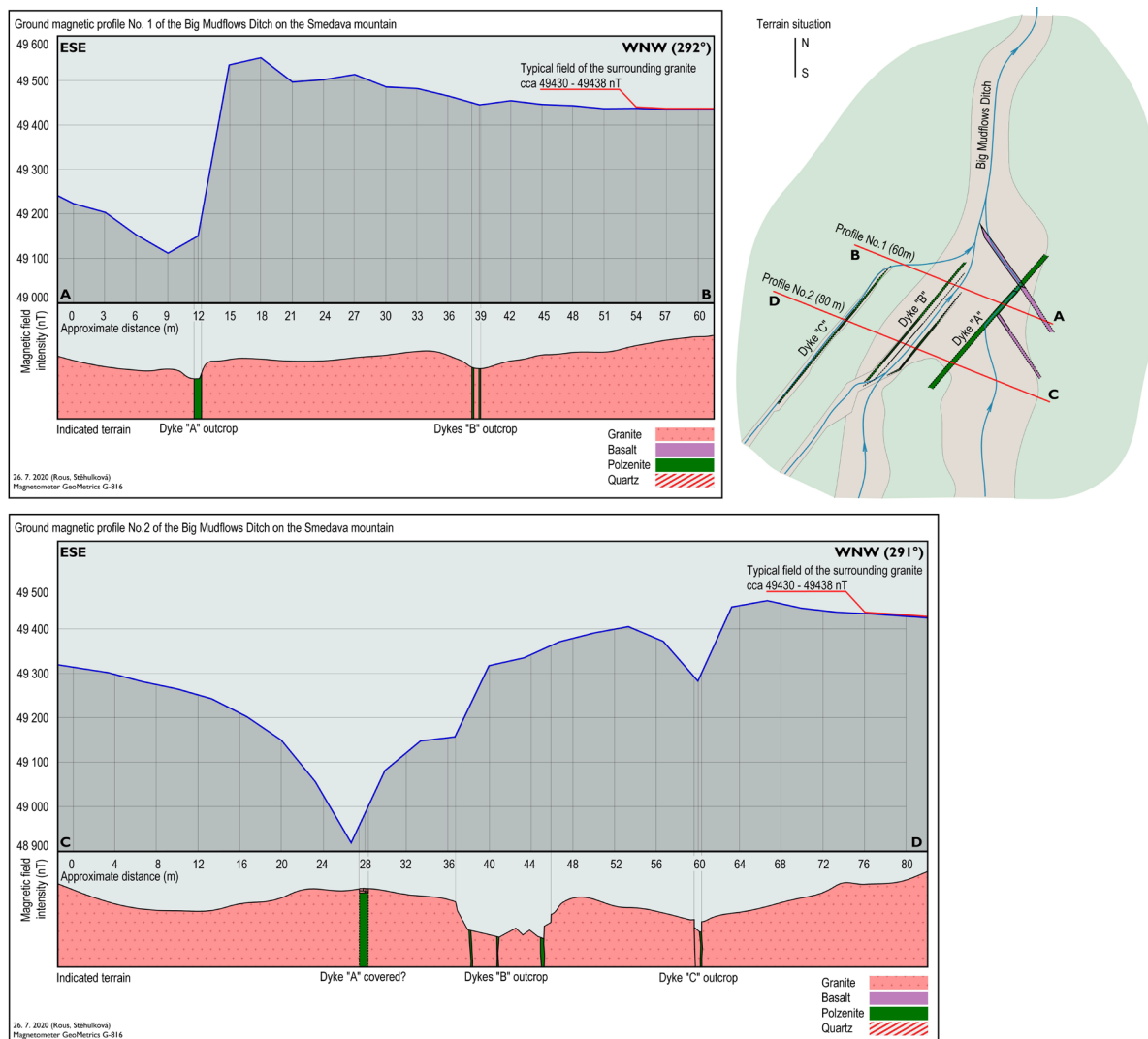
Obr. 4. Magnetometrie žilných těles na Smédavské hoře.
